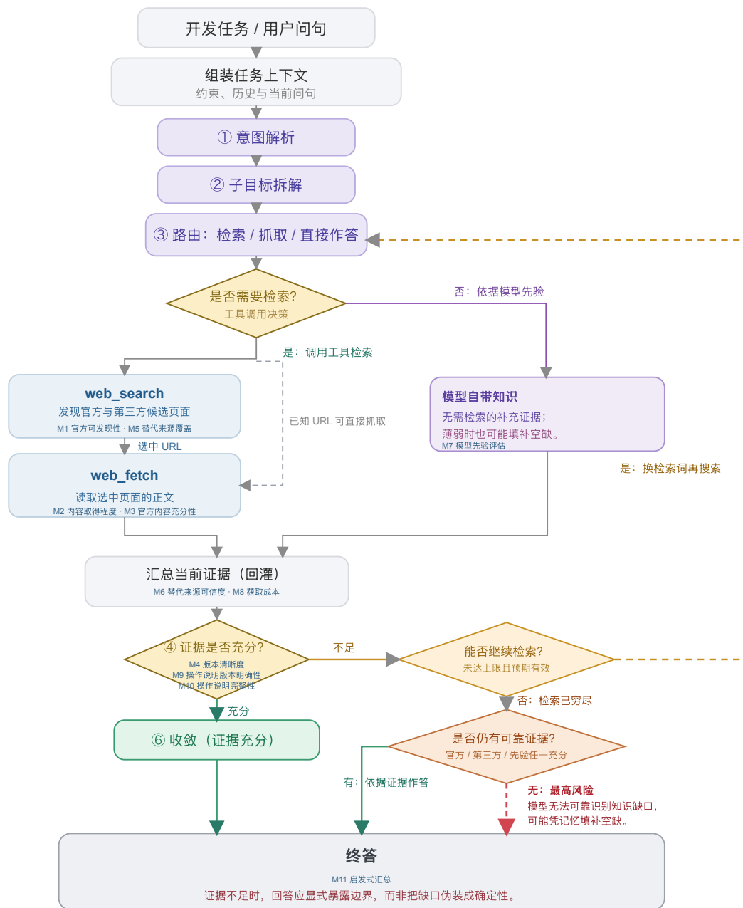
图 1 Agent 以任务与上下文为起点，经由意图解析、子目标拆解和路由判断，选择检索或模型先验；检索分支依次搜索、选取 URL、抓取正文或直接抓取已知 URL，再汇总证据并判断充分性。证据不足时可重试；检索穷尽时会区分是否仍有可靠证据。
