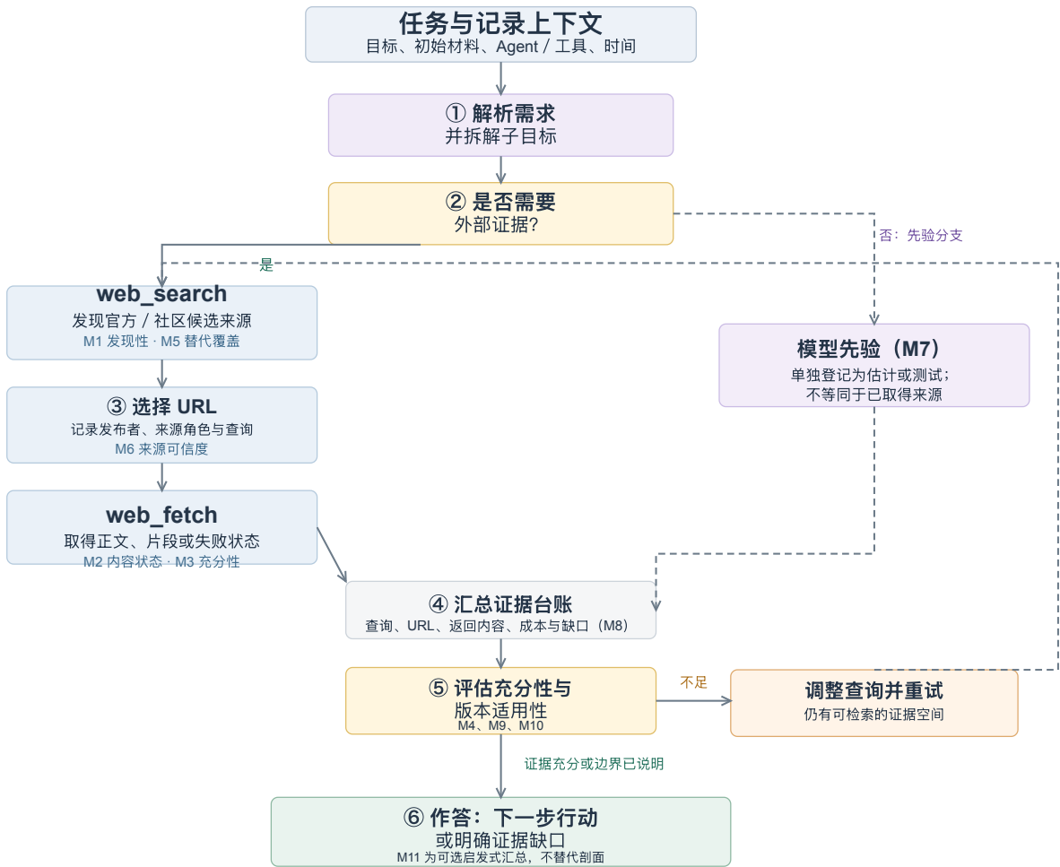
图 1 Agent 以任务与上下文为起点，经历检索、选择 URL、获取正文、汇总证据和充分性 / 版本检查；不足时精化查询并重试，先验知识保持为独立分支。
