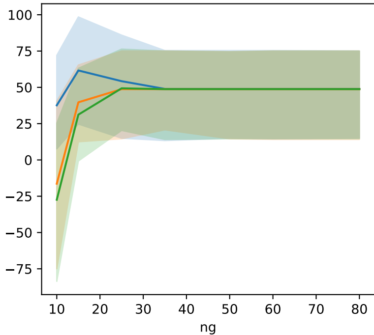
Lunar Lander-ES
