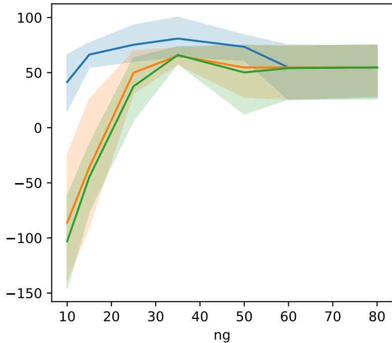
Lunar Lander-ES
