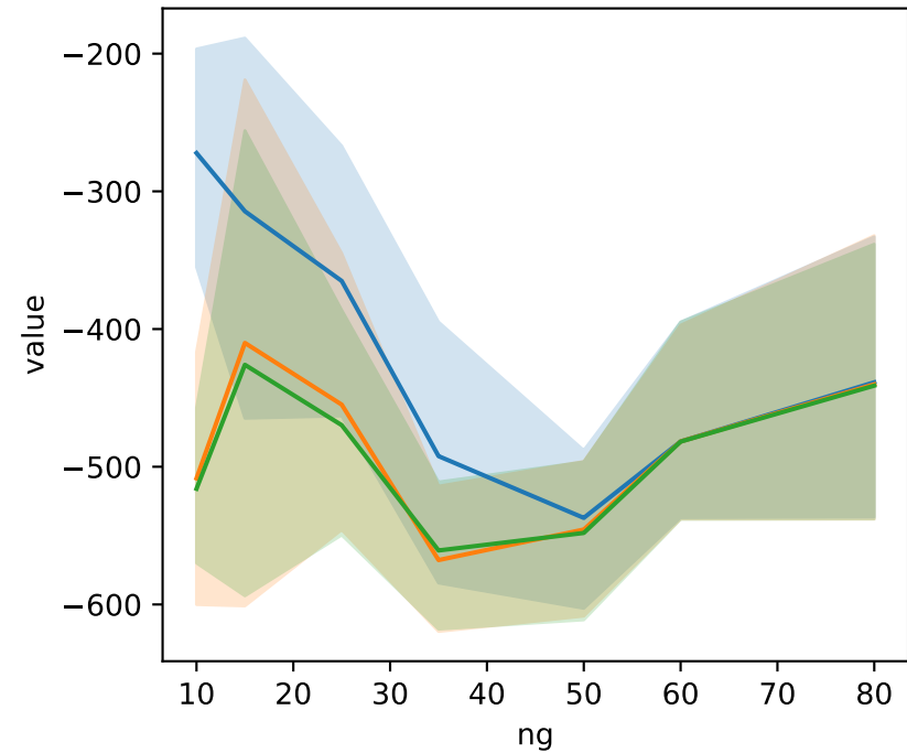
Lunar Lander-ES
