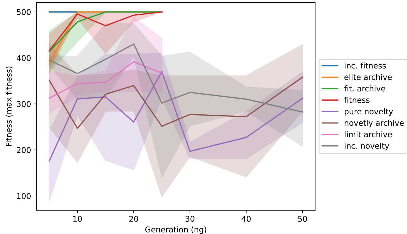
Cartpole-ES
