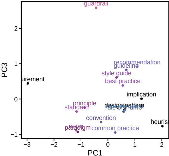
PCA Space: PC1 vs PC3
