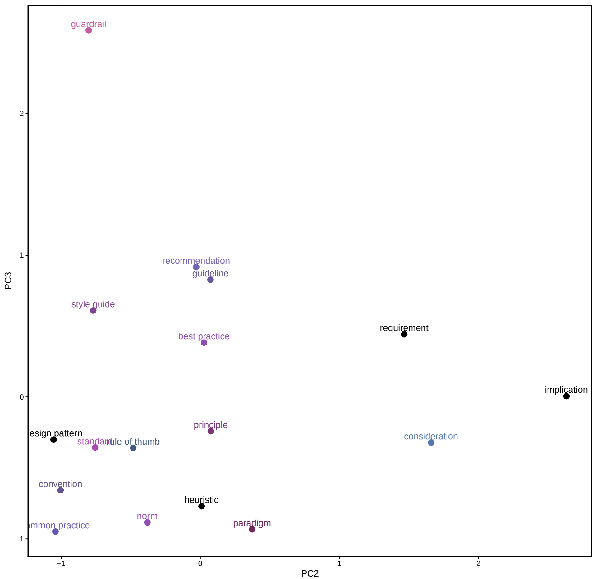
PCA Space: PC2 vs PC3
