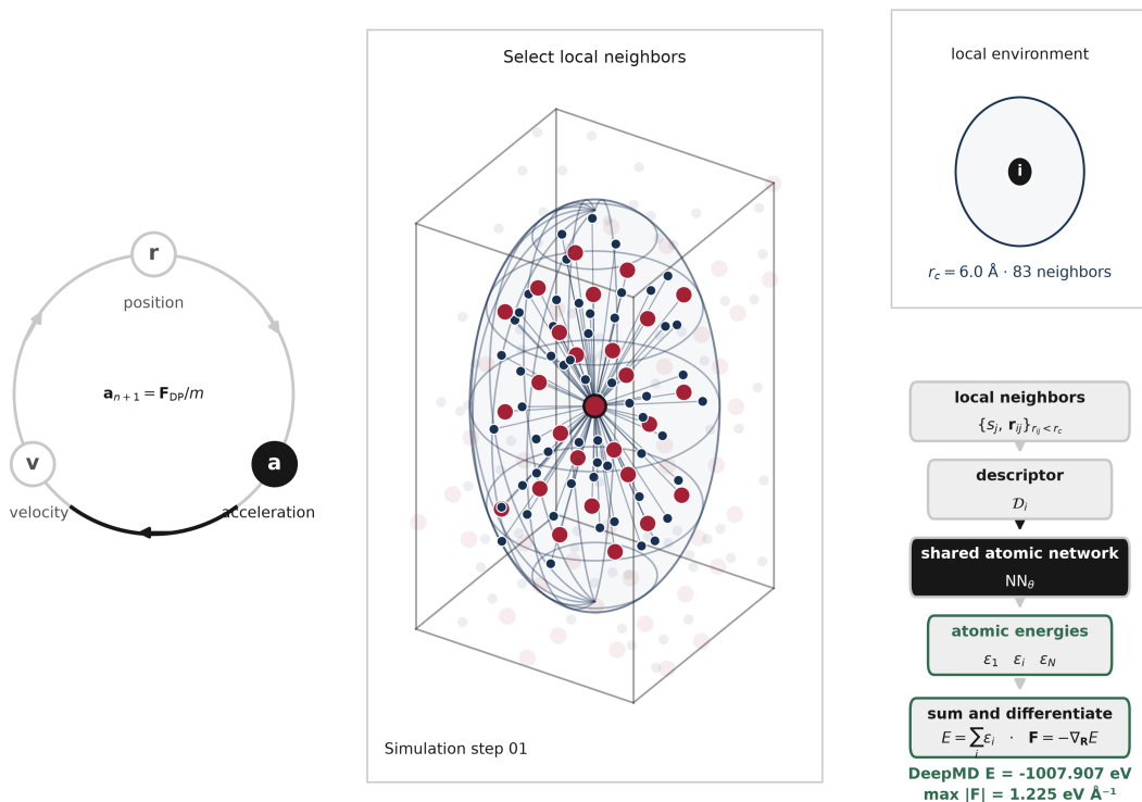
图 4: Deep Potential MD: 局域邻域经过共享模型汇总成能量和力，再返回外层积分器。真实三维盒、周期结构、双色化学键、截断球和原子中心向量应由同一结构渲染体系生成。
