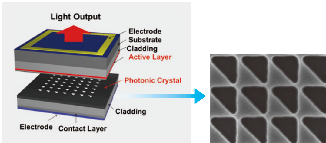
SEM image
