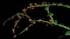
EGFP (dendrite) — EYFP (synapse) XY.
