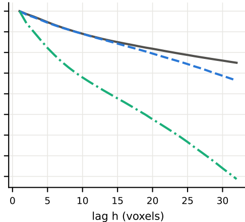
meander-oxbow — y
