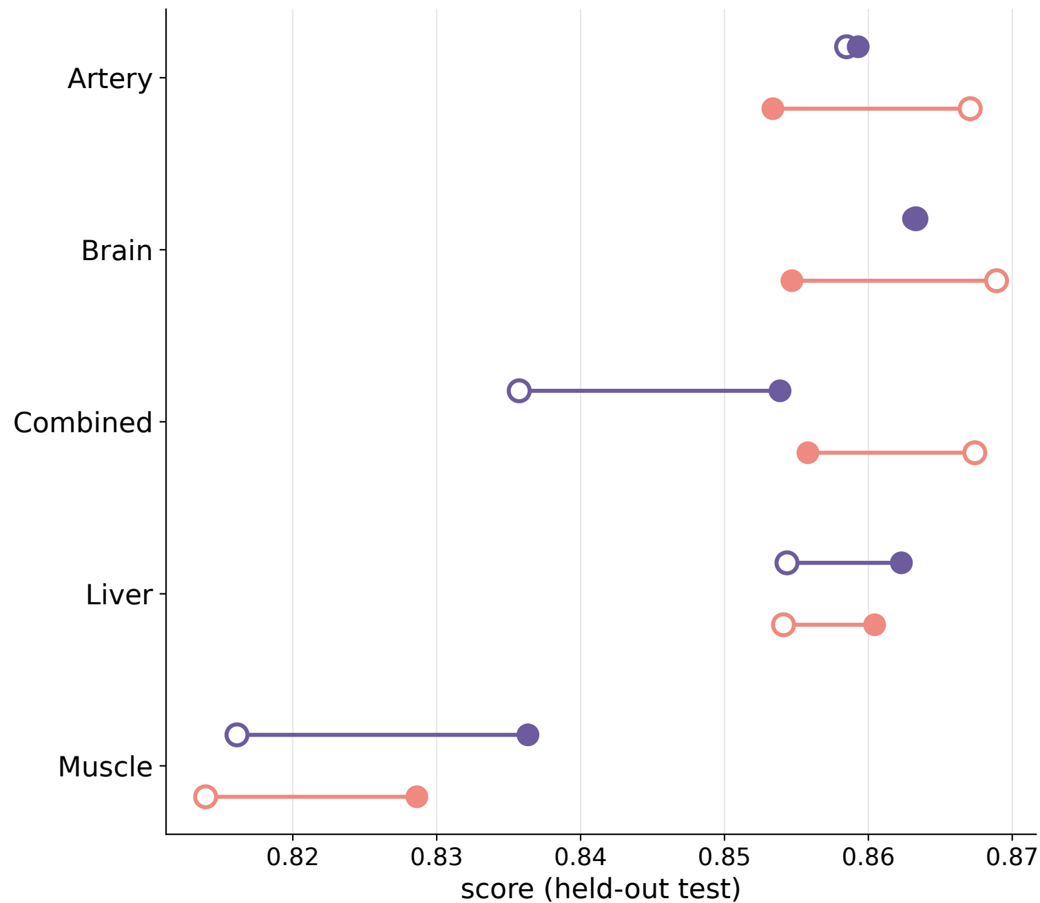
Test F1
