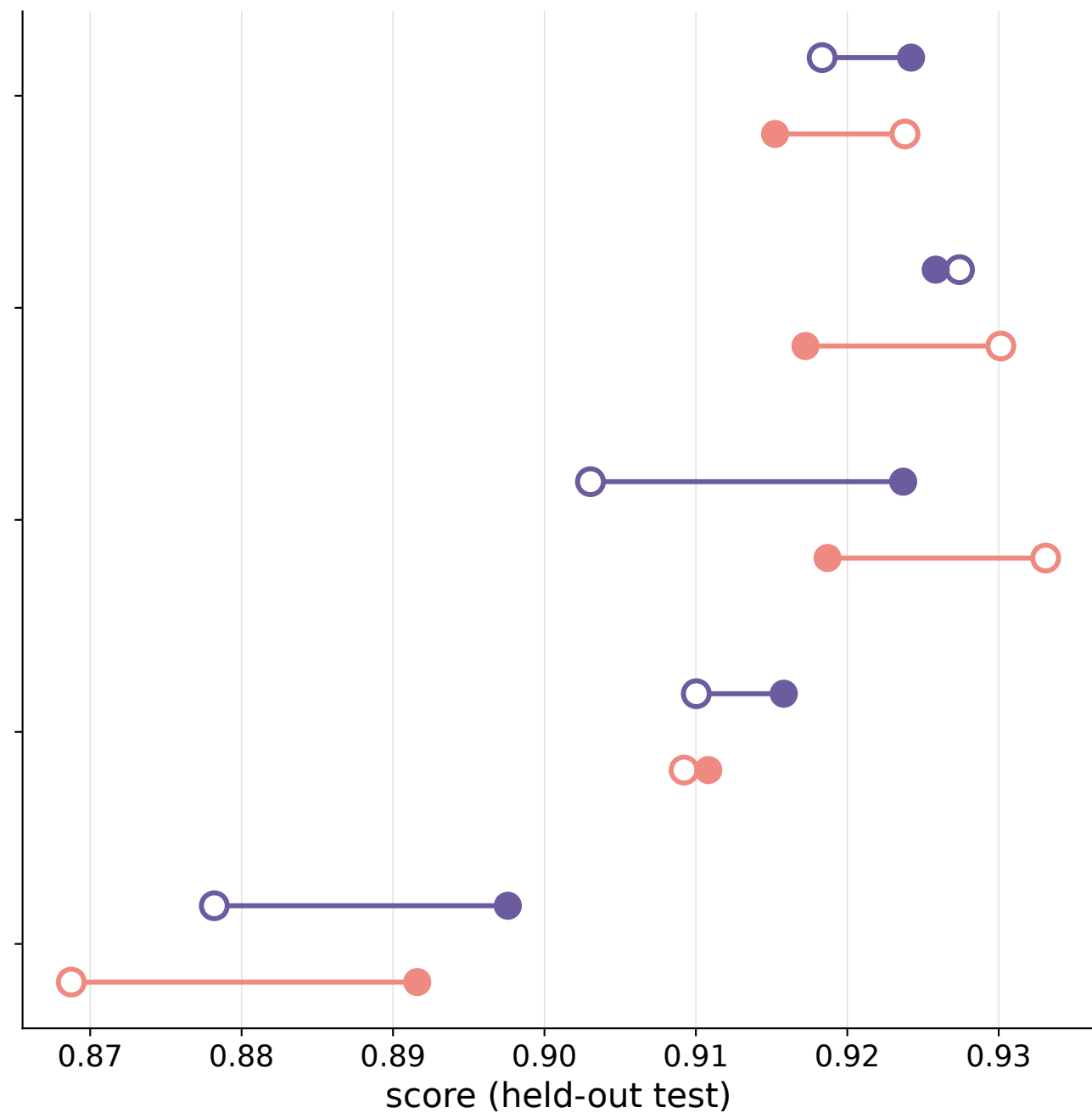
Test AUROC
