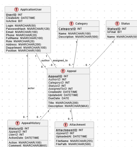
Рисунок 2 – ER-диаграмма базы данных
