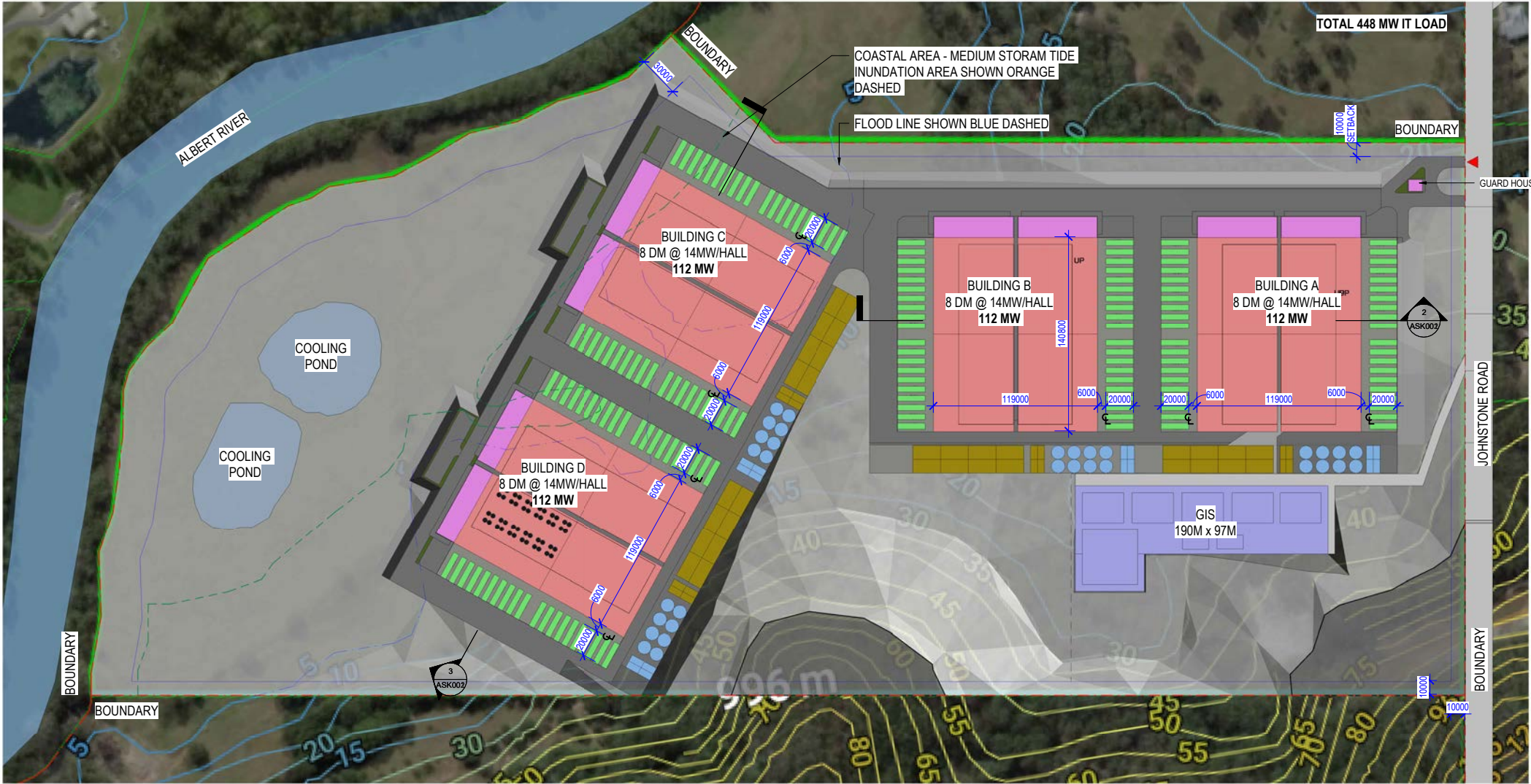
1 SITE PLAN_OP1 1:2000
