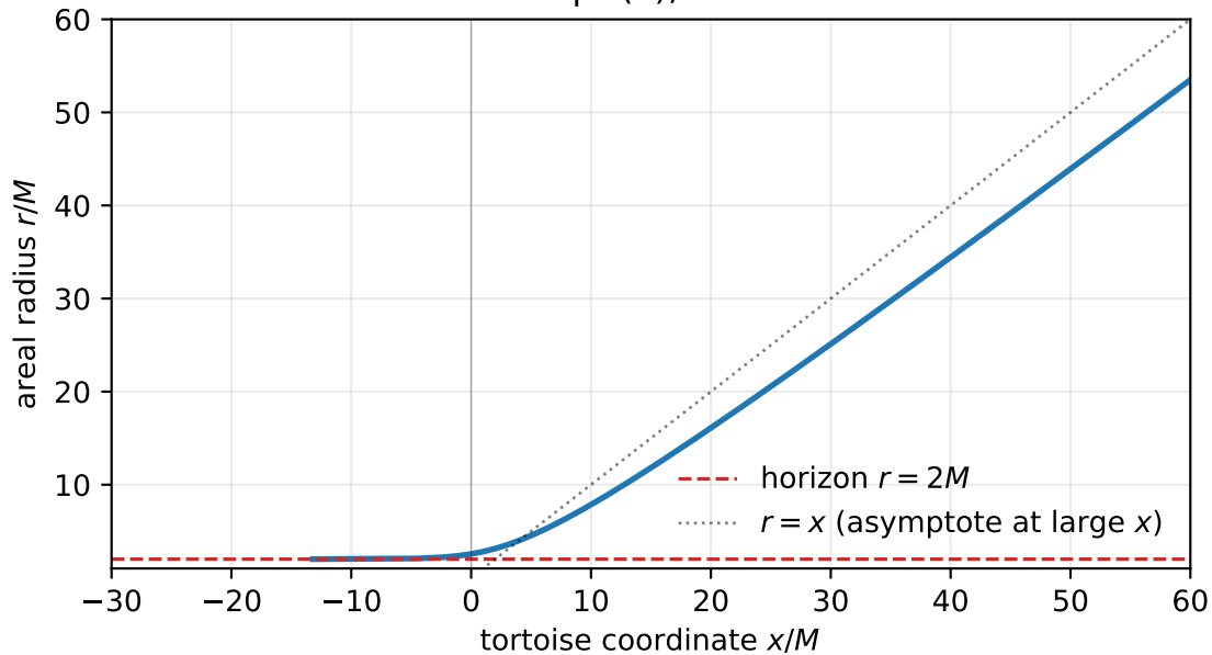
Tortoise map r(x) , Schwarzschild
