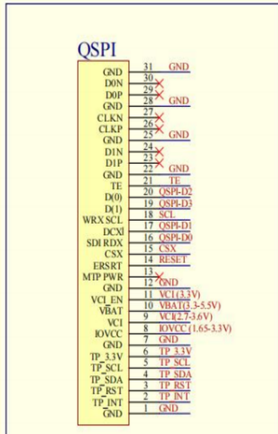
QSPI接口参考接线图
