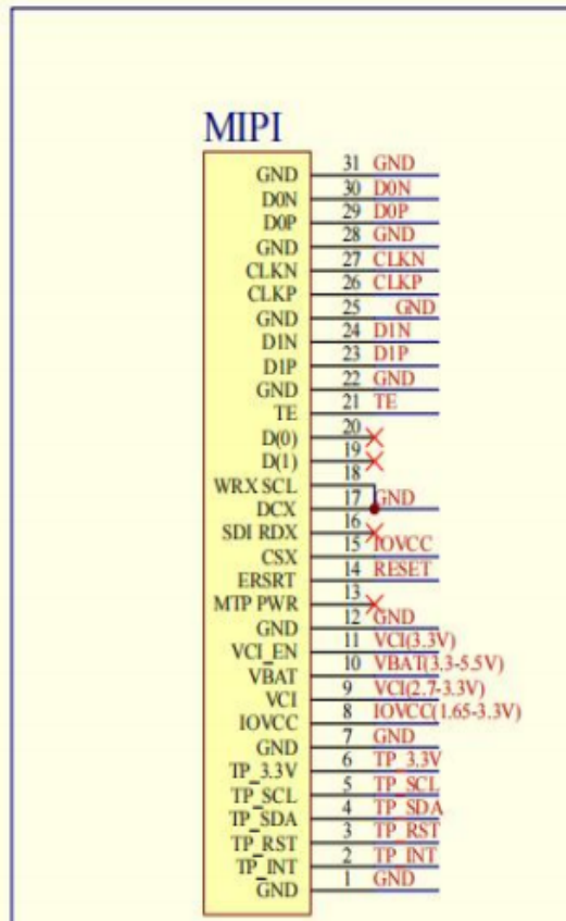
mipi接口参考接线图
