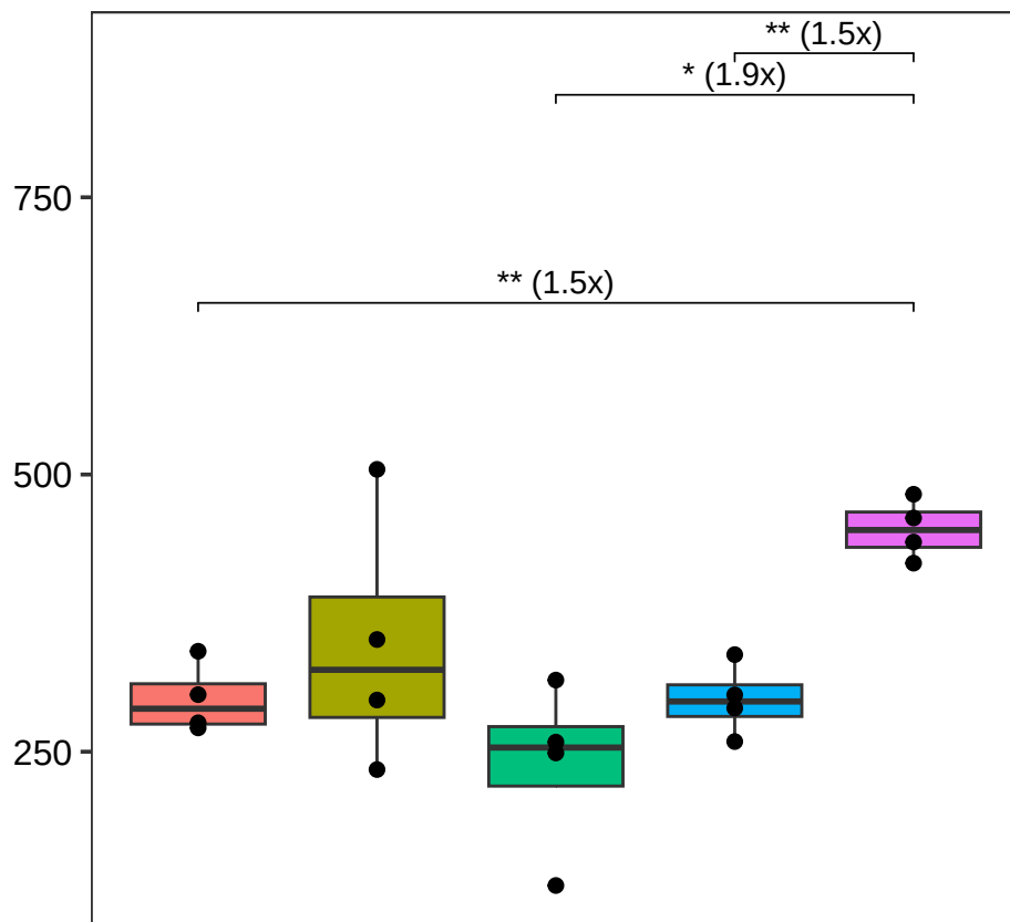
TcmE
