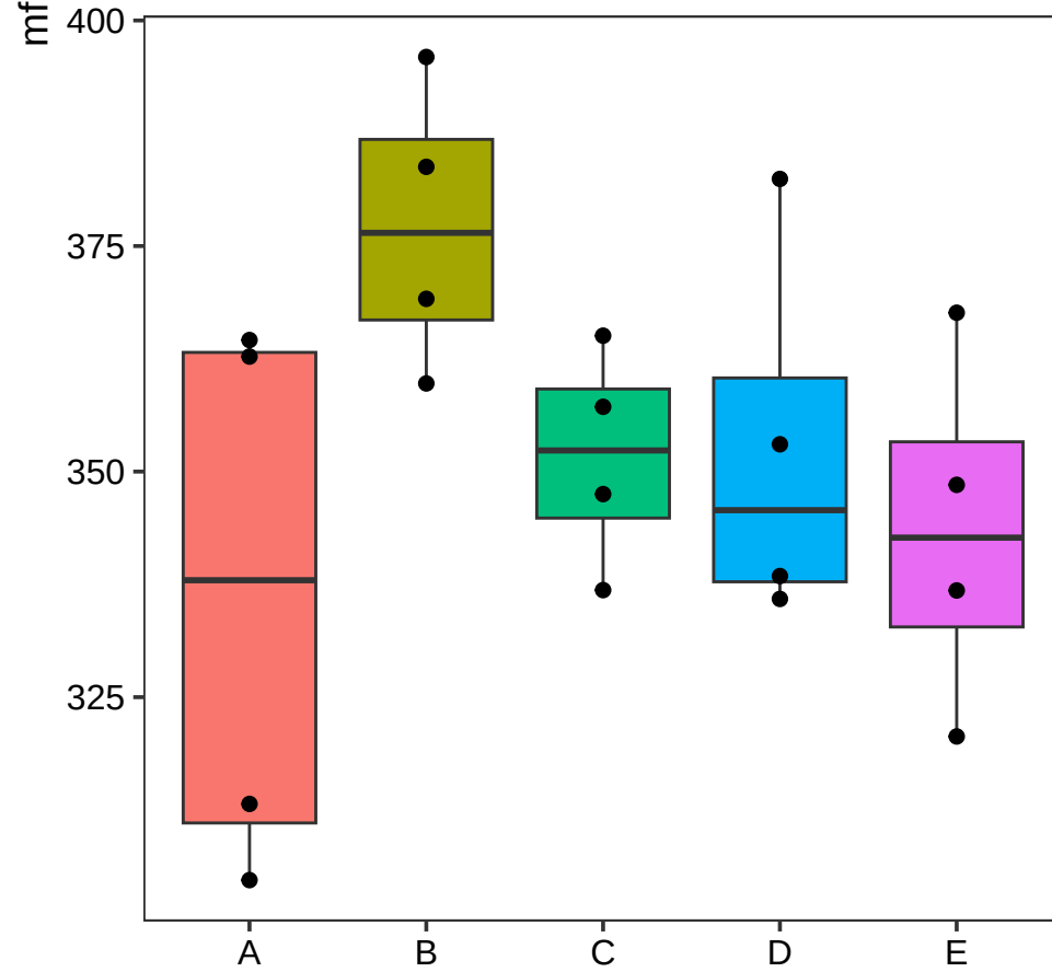
Tcf1Pos
