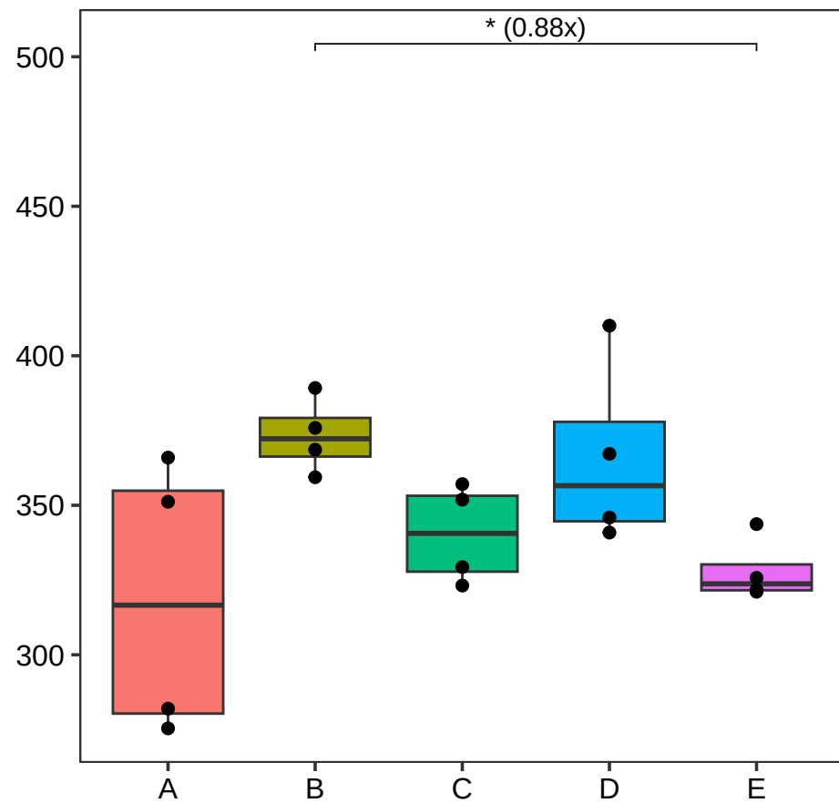
ToxPos
