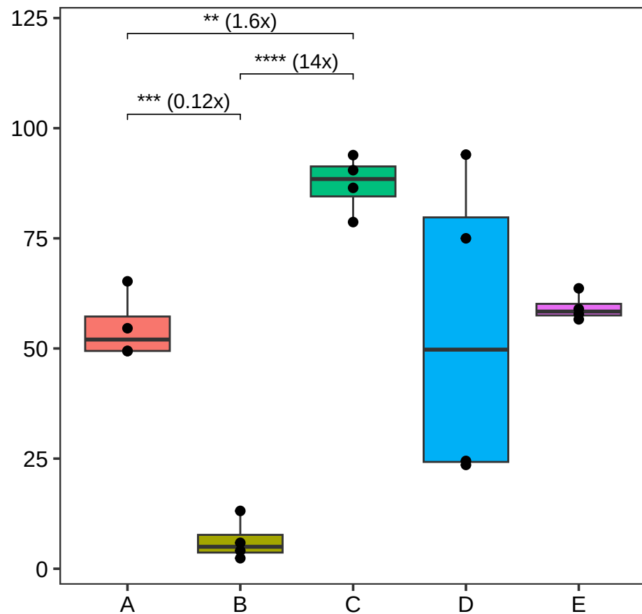
ToxPos
