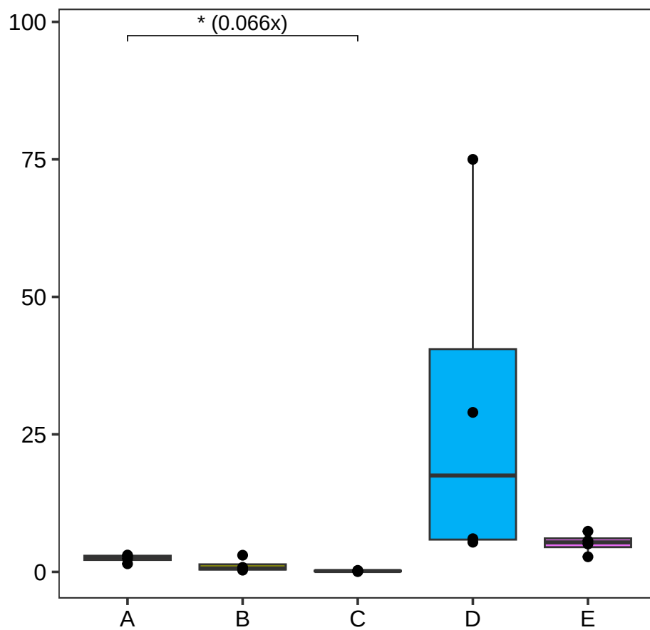
Tcf1Pos
