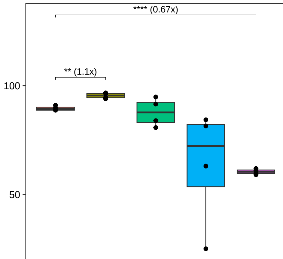
CXCR6Pos
