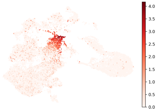
GP9
