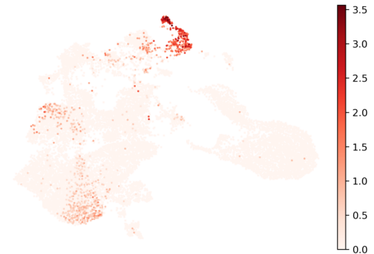
EMCN
