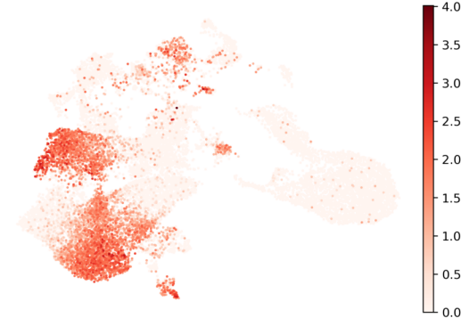
HOPX
