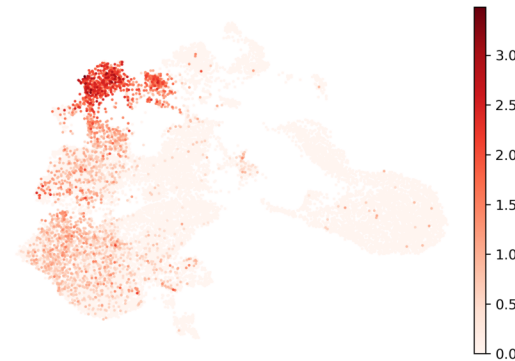
CSF1R
