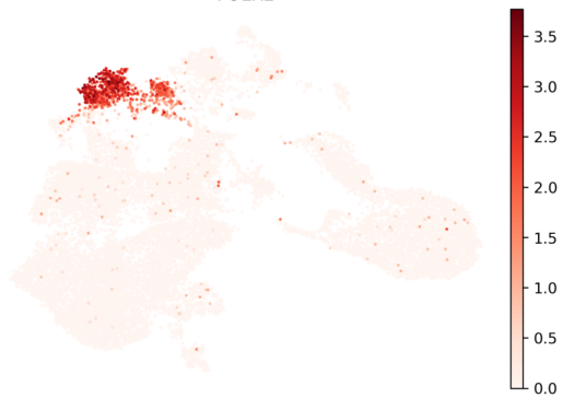
FOLR2
