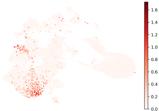
AVP
