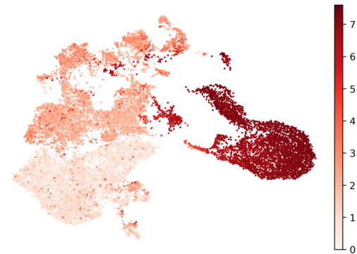
HBA1
