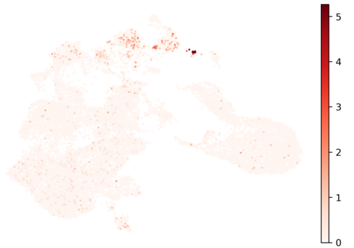
TTR
