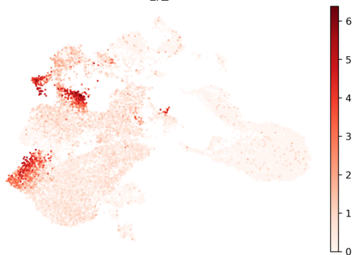
LYZ
