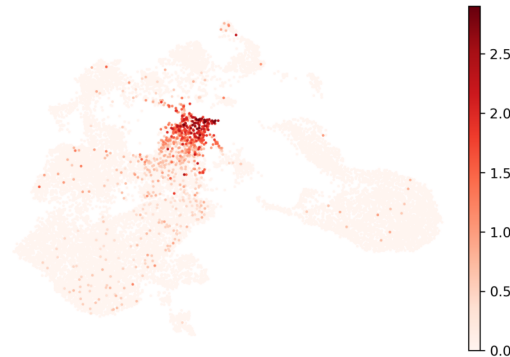
GP1BA
