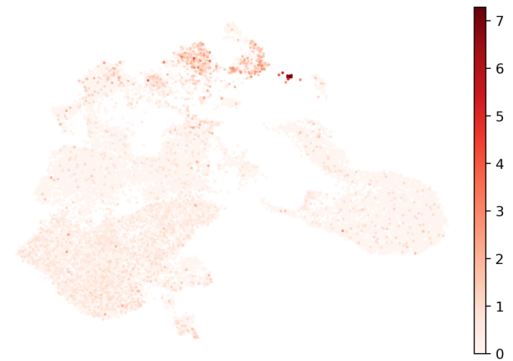
ALB
