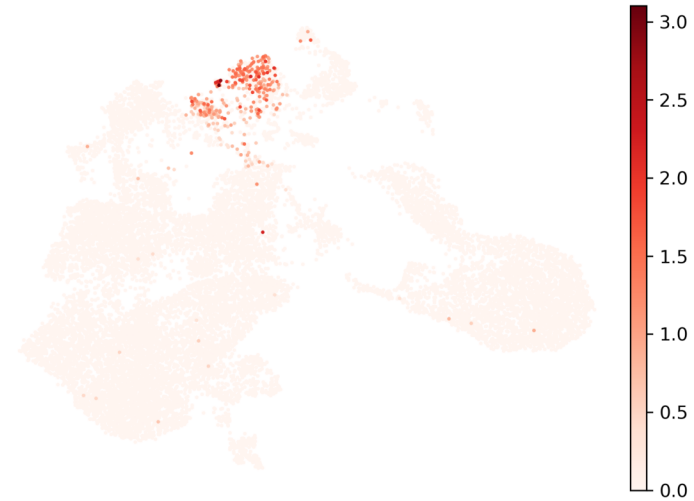
PDGFRA
