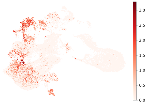
IRF8
