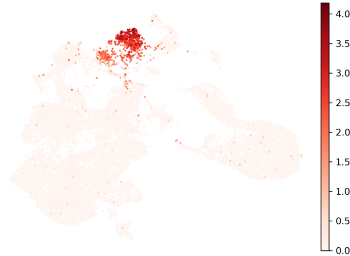
DCN
