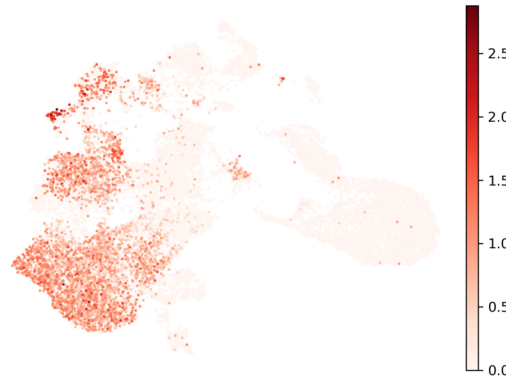
CSF3R
