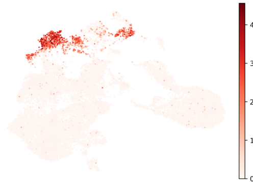
CD14
