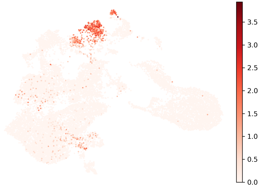
PDGFRB
