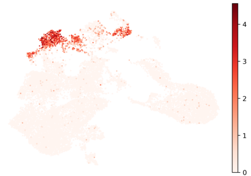
CD14
