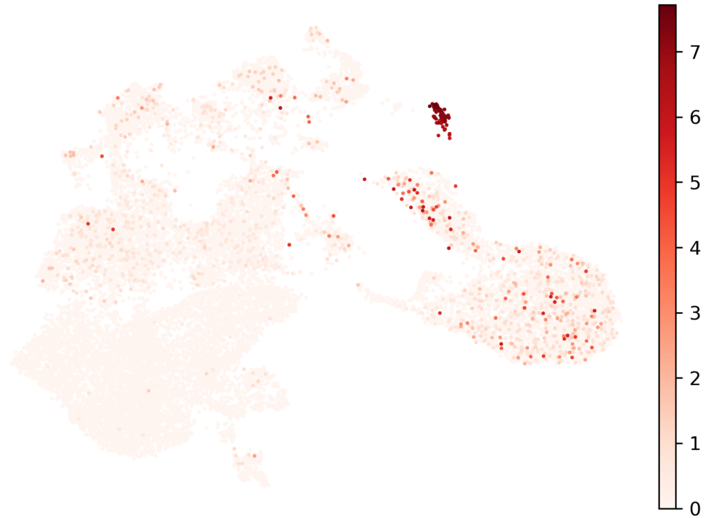
HBE1
