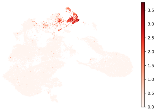
KDR
