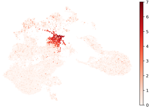
PF4
