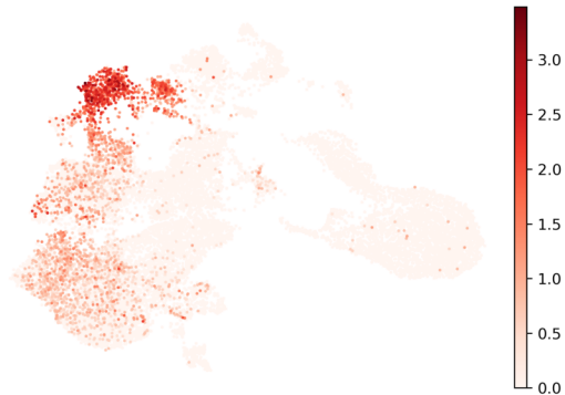
CSF1R
