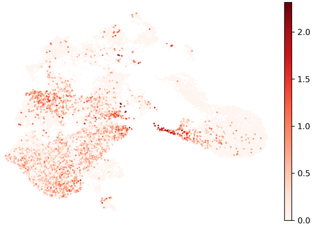
EPCAM
