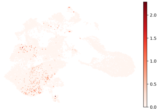
PRDM16
