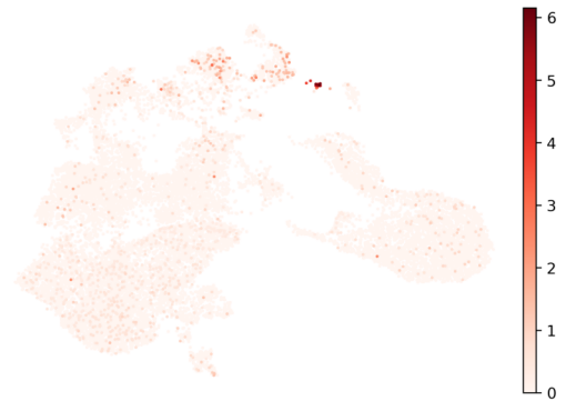
AFP
