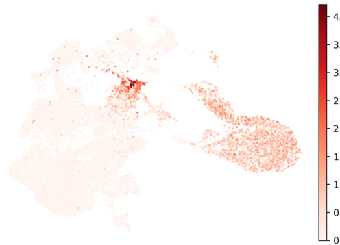
TUBB1
