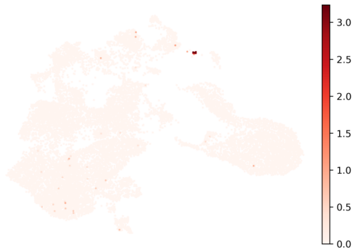
FGA
