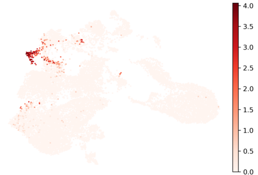
FCN1
