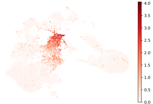
ITGA2B
