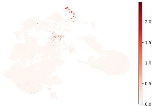
VWF
