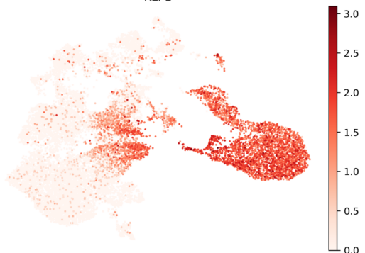
KLF1
