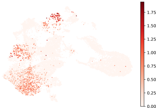
PROM1
