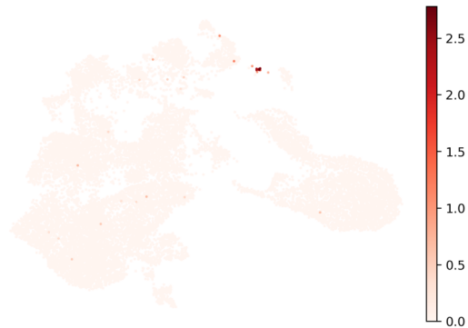
HPX
