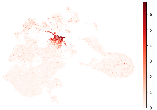
PPBP
