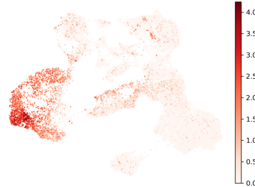
CSF3R
