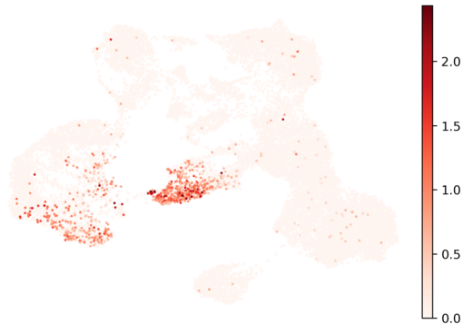
IRF8
