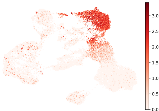
GP1BA
