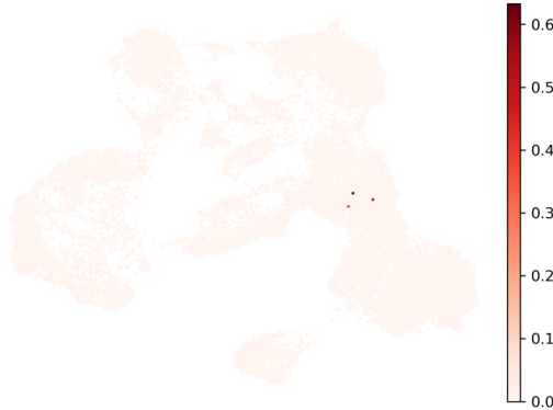
POU5F1
