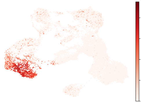
CD14
