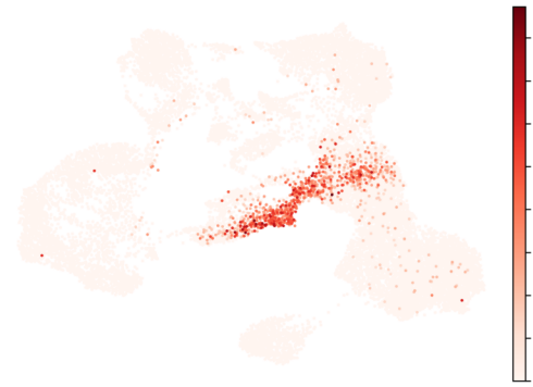
CD34
