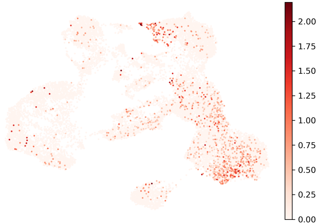
ACTA2
