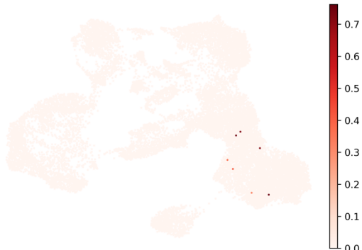
FGA
