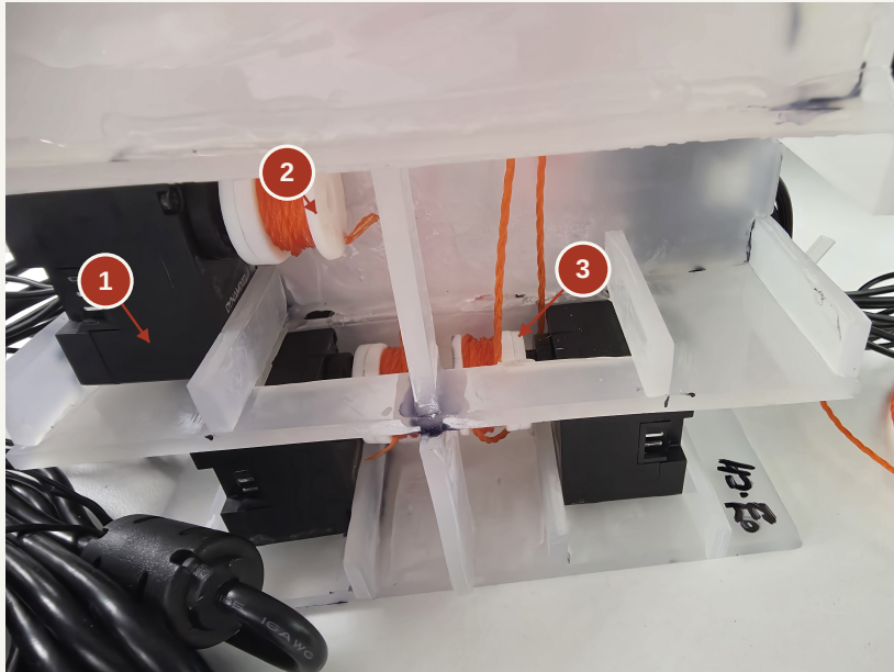
구동부 내부: 모터·스푼·텐던 연결
