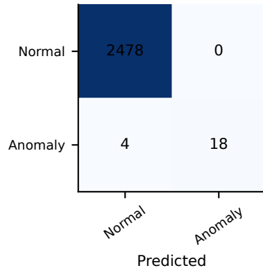
PCA Reconstruction
