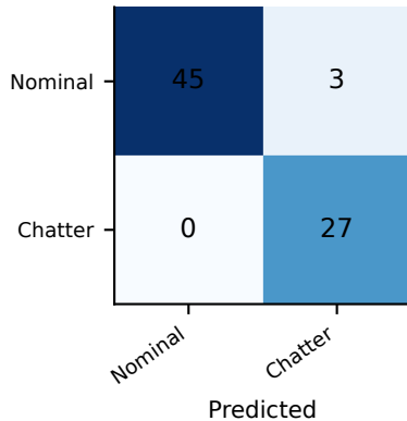
PCA reconstruction
