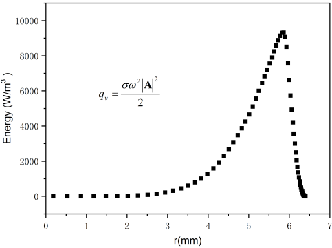
图 5-1 内热源沿径向的分布
