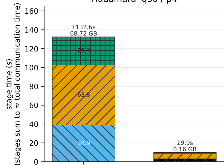
Hadamard q30 / p4
