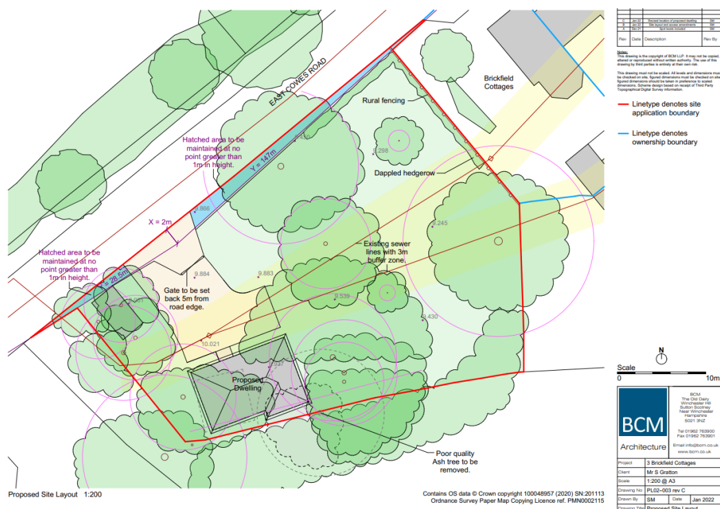
Plan no. PL02-003 Rev. C
