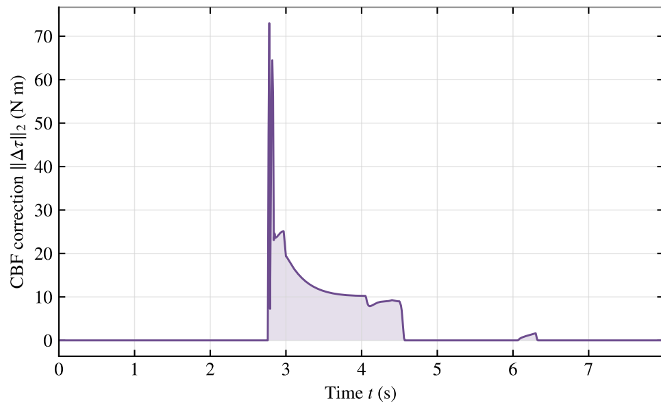
(d) CBF control intervention
