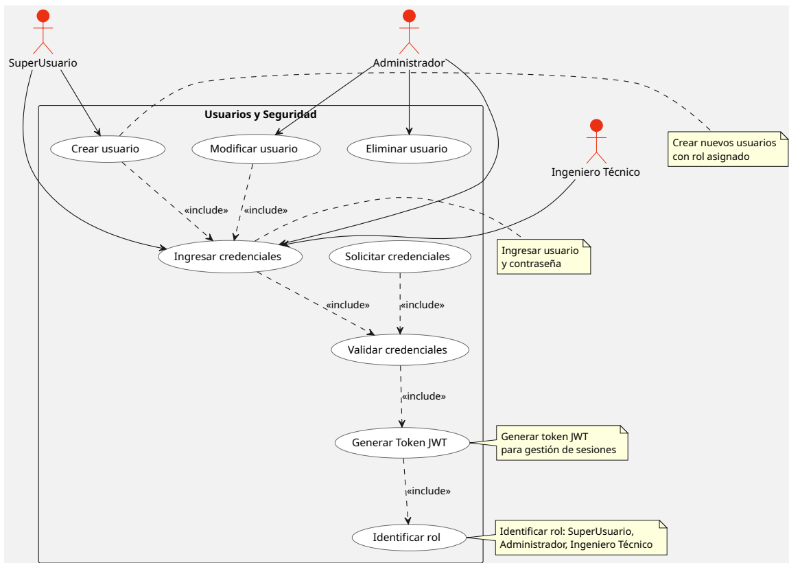
Figure 10: CU - Usuarios y Seguridad
