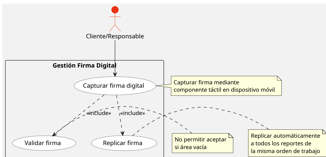
Figure 5: CU - Gestión de Firma Digital
