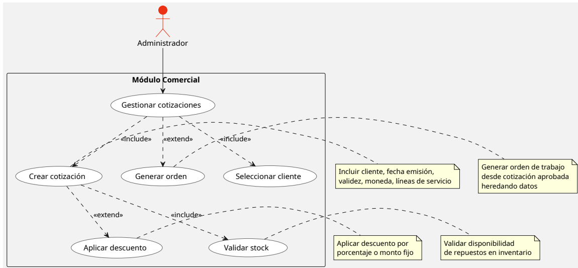
Figure 9: CU - Módulo Comercial
