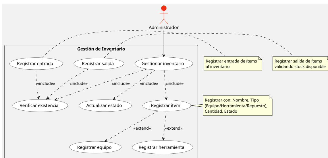
Figure 7: CU - Gestión de Inventario
