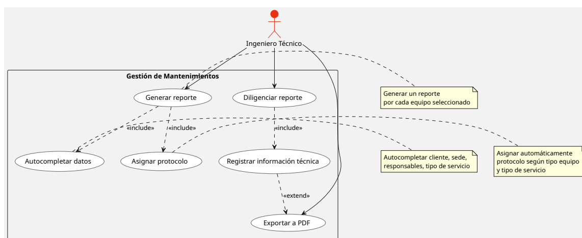
Figure 4: CU - Gestión de Mantenimientos
