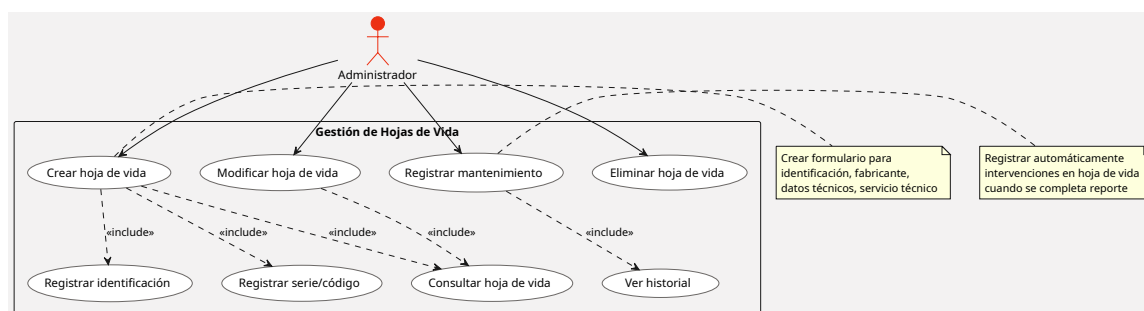
Figure 6: CU - Gestión de Hojas de Vida
