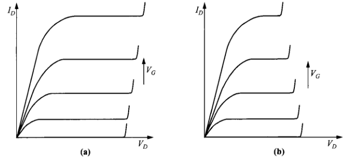
Figura 33: Datos experimentales que muestran que la tensión de ruptura del drenador (a) aumenta con V_{GS} , en JFET de Si, pero (b) disminuye con V_{GS} , en MESFET de GaAs (Sze et al., 2021).
