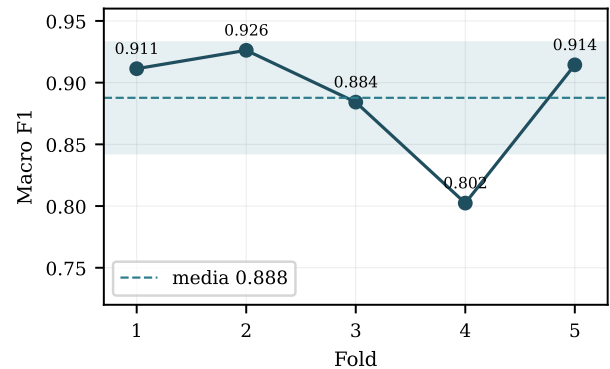
Figura 9. Macro F1 por fold en la validación cruzada. La caída del fold 4 (0,80) refleja la sensibilidad de la métrica macro a las clases minoritarias y justifica reportar la CV en lugar de un split único.
