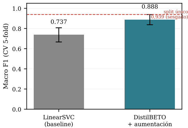
Figura 5. Macro F1 bajo validación cruzada 5-fold. DistilBETO supera al baseline LinearSVC con margen robusto. La línea punteada marca el Macro F1 del split único (0,939), optimista por el sesgo de selección de checkpoint.
