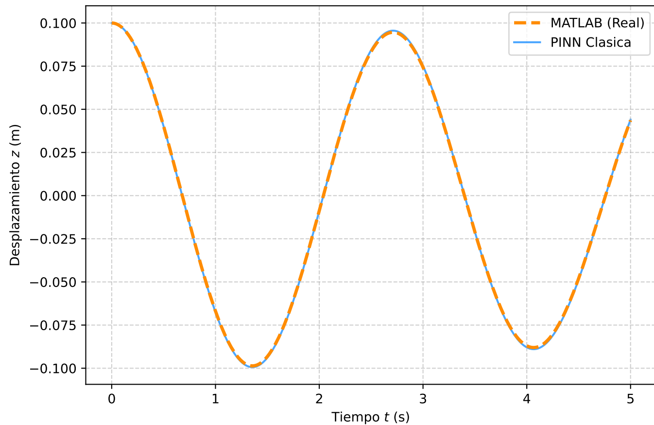
Movimiento Translacional z(t) - [0 a 5s]
