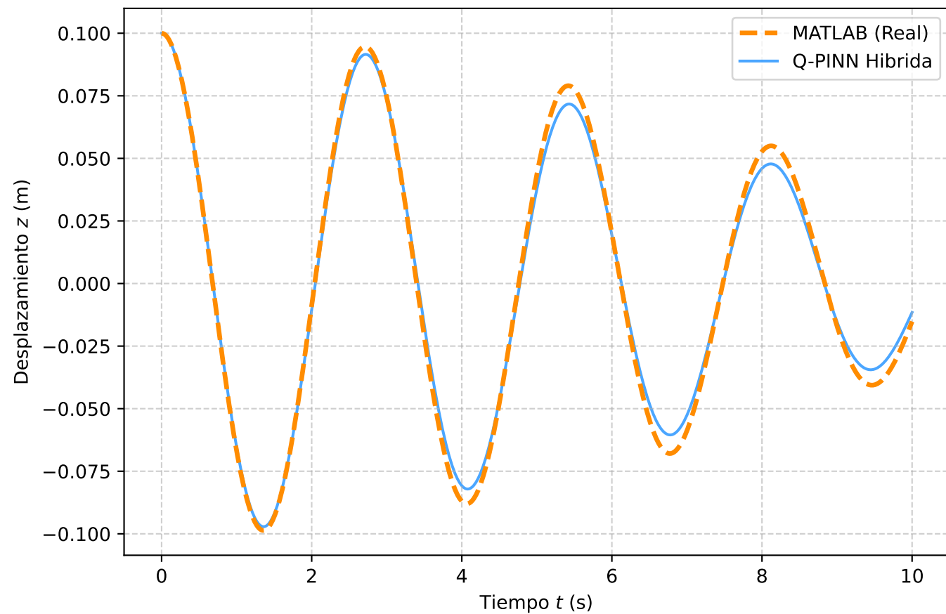
Movimiento Translacional z(t) - [0 a 10s]
