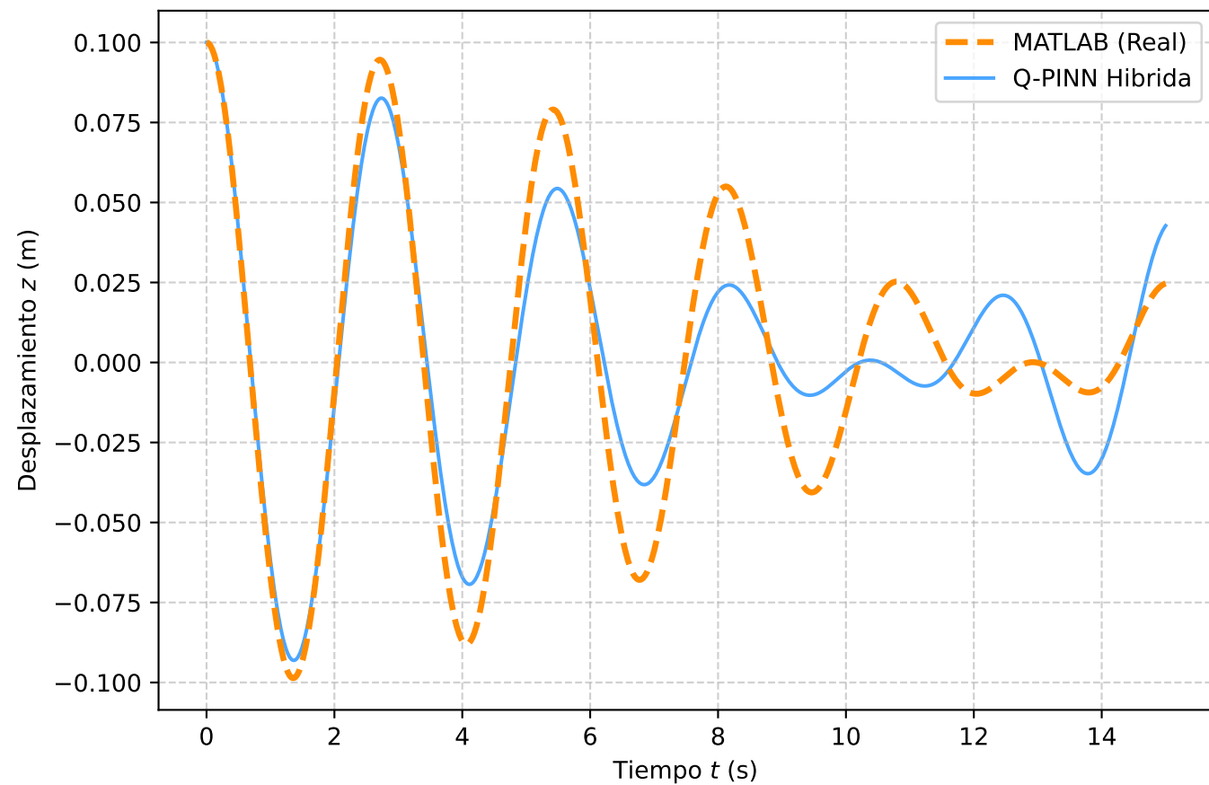
Movimiento Translacional z(t) - [0 a 15s]
