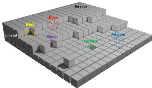
Fig. 5. Sitios de adsorción del modelo SOS.
