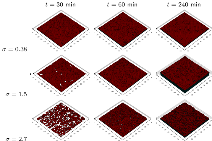
Fig. 15. Snapshots del modelo 3D isotrópico (red 80 \times 80 ).
