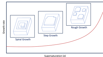
Fig. 4. Regímenes de crecimiento según la sobresaturación \sigma .
