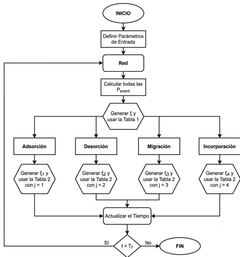
Fig. 12. Diagrama de flujo del algoritmo kMC.
