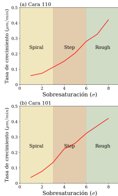
Fig. 13. Tasa de crecimiento vs. \sigma , caras (110) y (101).
