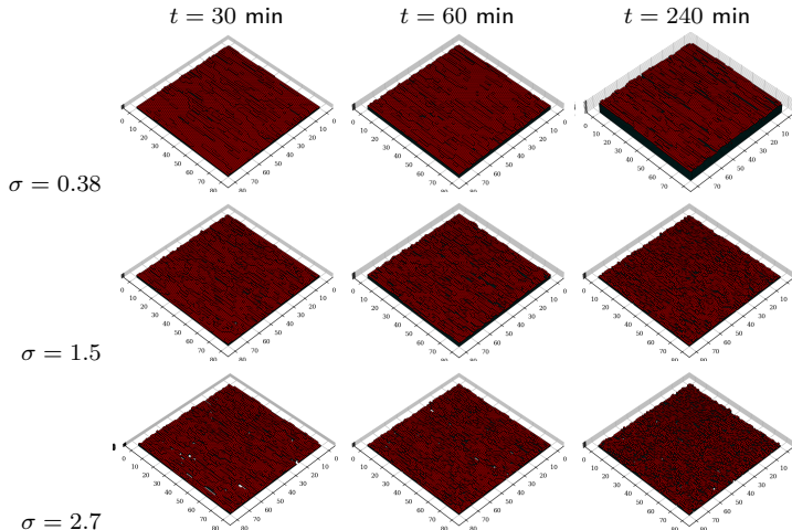
Fig. 9. Snapshots del modelo 3D anisotrópico (red 80 \times 80 ).
