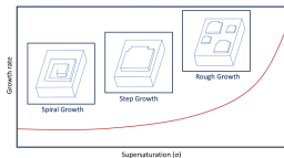
Fig. 4. Regímenes de crecimiento según la sobresaturación \sigma .
