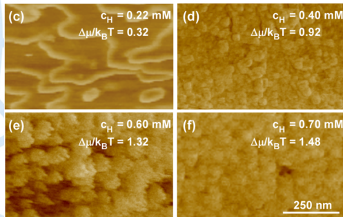
Fig. 10. AFM (modo de fase) a distintas \sigma .
