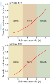
Fig. 13. Tasa de crecimiento vs. \sigma , caras (110) y (101).
