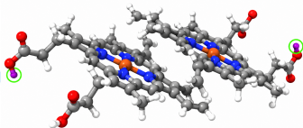
Fig. 3. O externos saturados con H (evita el colapso de los carboxilos en vacío). Relajación L-BFGS en dos etapas: H añadidos \rightarrow todos los átomos.
