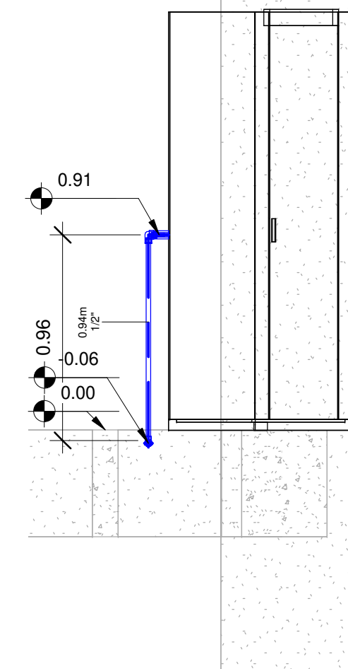
1 Aparato critico 1 : 25
