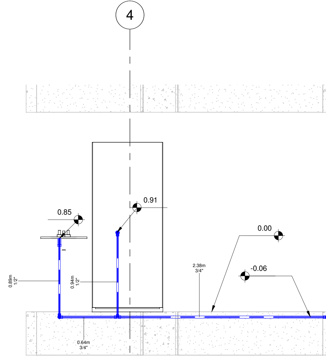
3 Red agua fria aparato critico 1 : 25
