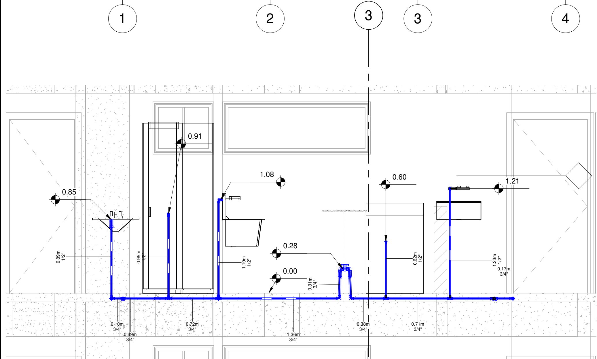
2 Distribucion red agua fria 1 : 25
