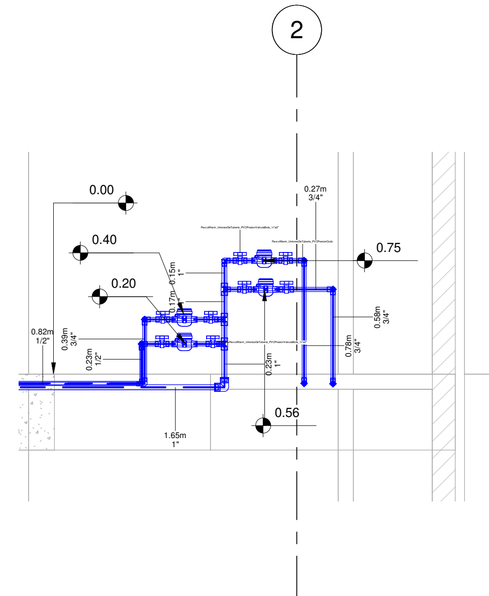
4 Medidores 1 : 25
