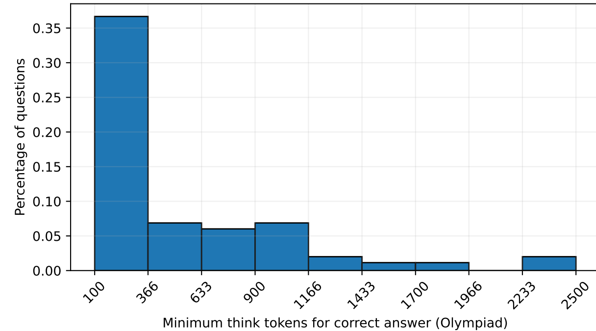
Olympiad
