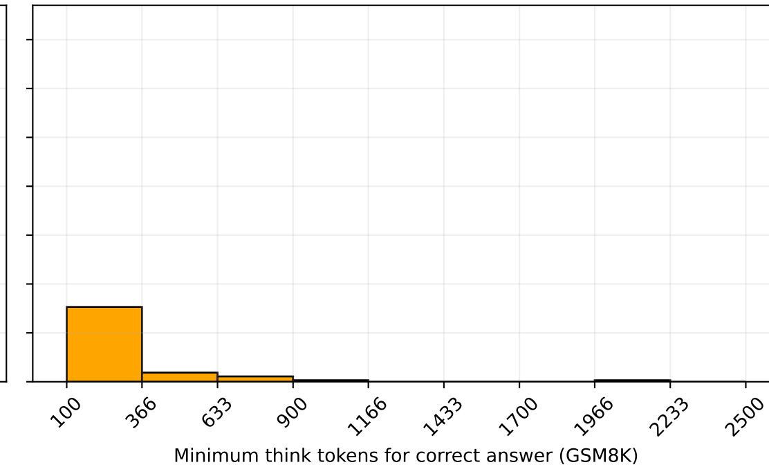
GSM8K
