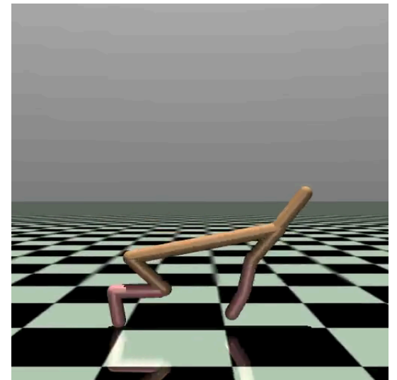
PPO
