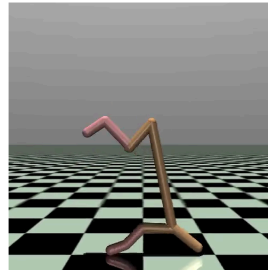
TRPO
