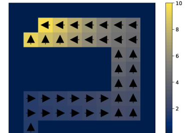
(d) IQL
