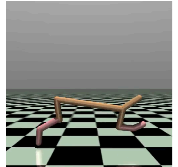
SAC
