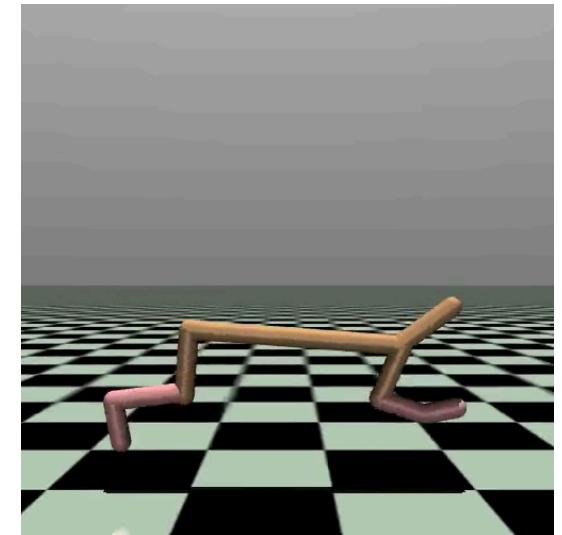
TD3
