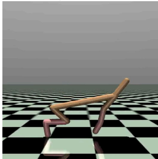
PPO
