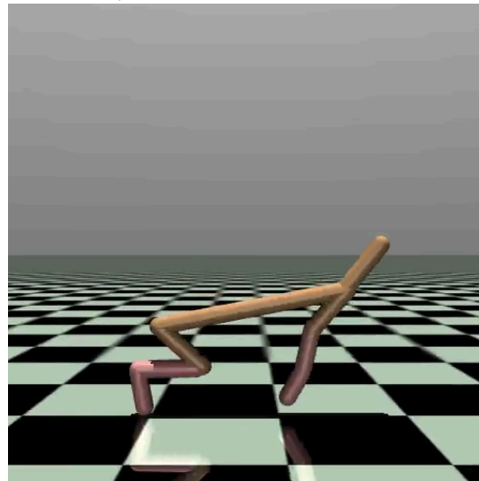
PPO
