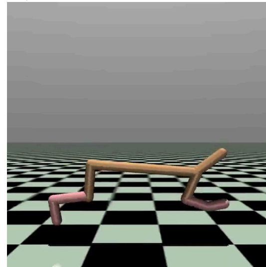
TD3
