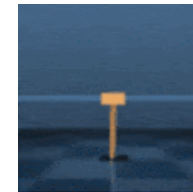
Sparse Cartpole
