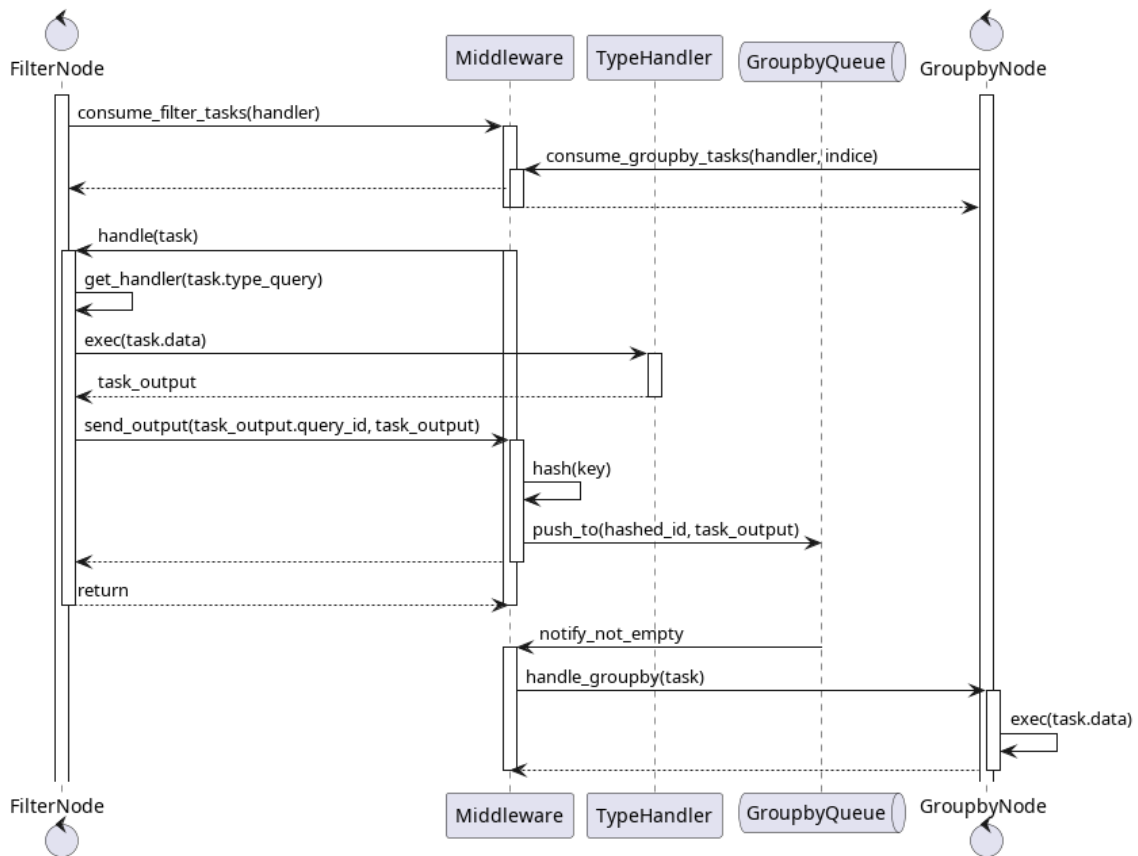
Figura 3: Diagrama de secuencia: Filter Node
