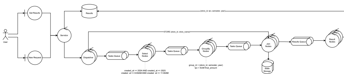
Figura 9: Diagrama de robustez consulta 3°
