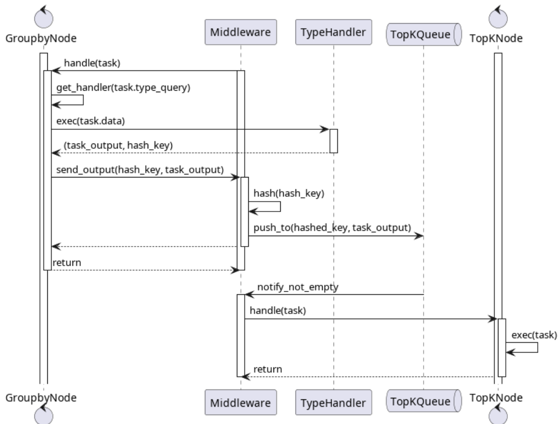
Figura 4: Diagrama de secuencia: GroupBy Node
