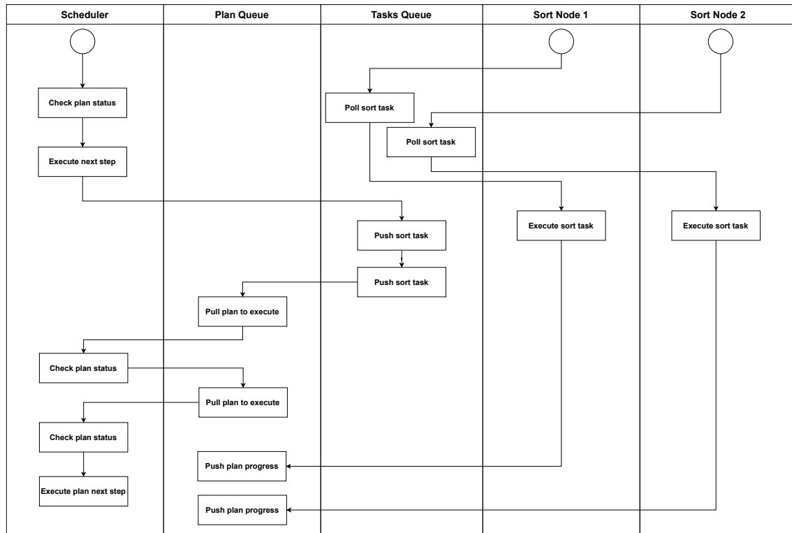
Figura 1: Diagrama de actividades
