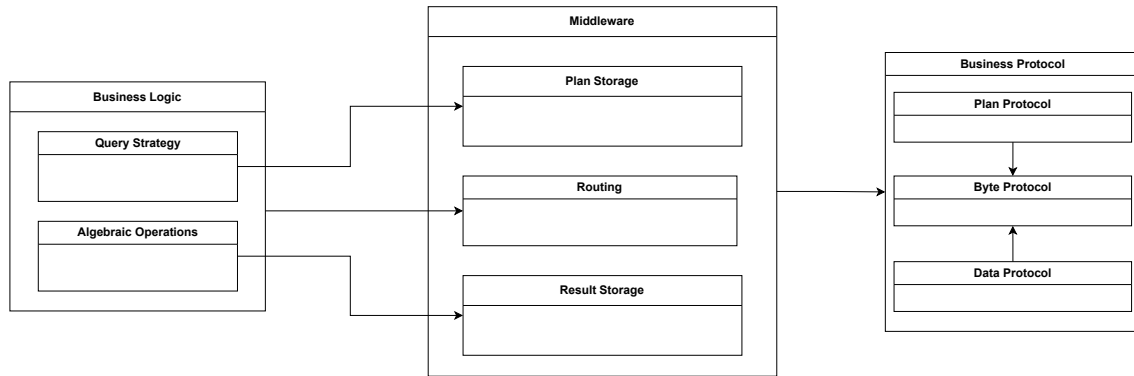
Figura 6: Diagrama de paquetes
