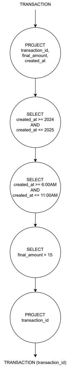
Figura 2: Diagrama DAG consulta 1°
