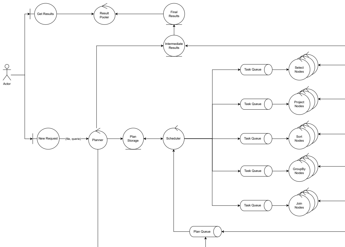
Figura 7: Diagrama de robustez
