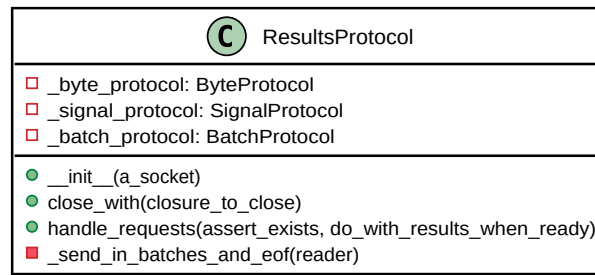
Figura 12: Diagrama de clase del protocolo del resultado
