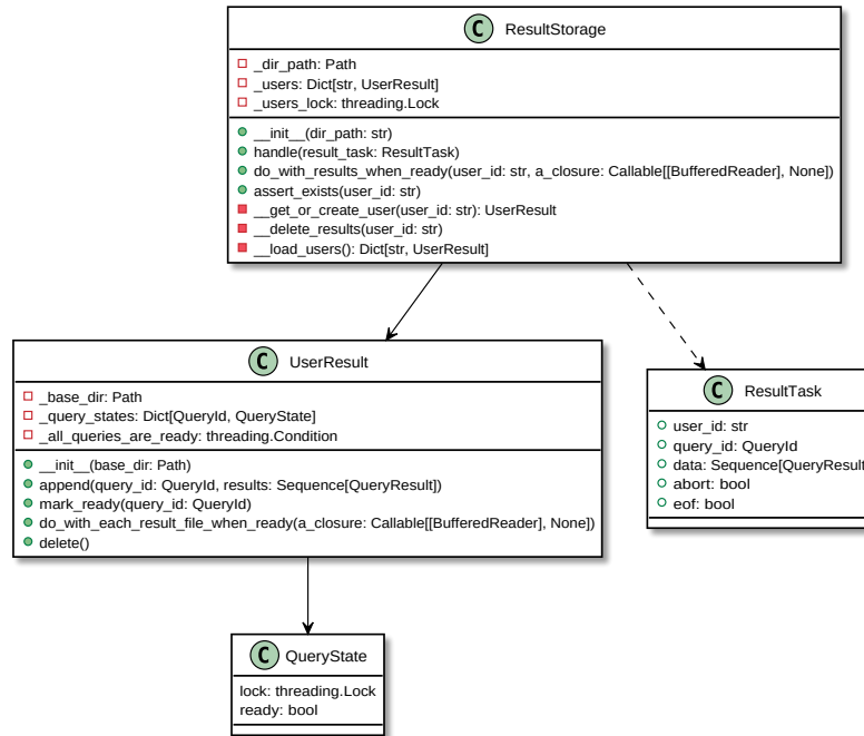
Figura 8: Diagrama de clases del almacenamiento de resultados
