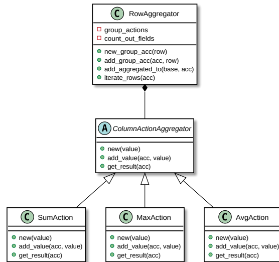
Figura 6: Diagrama de clases del nodo de agregación
