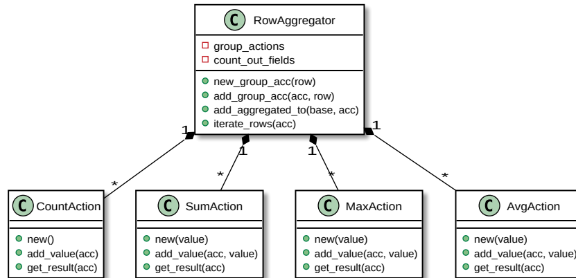
Figura 6: Diagrama de clases del nodo de agregación
