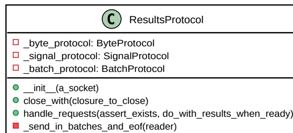
Figura 12: Diagrama de clase del protocolo del resultado
