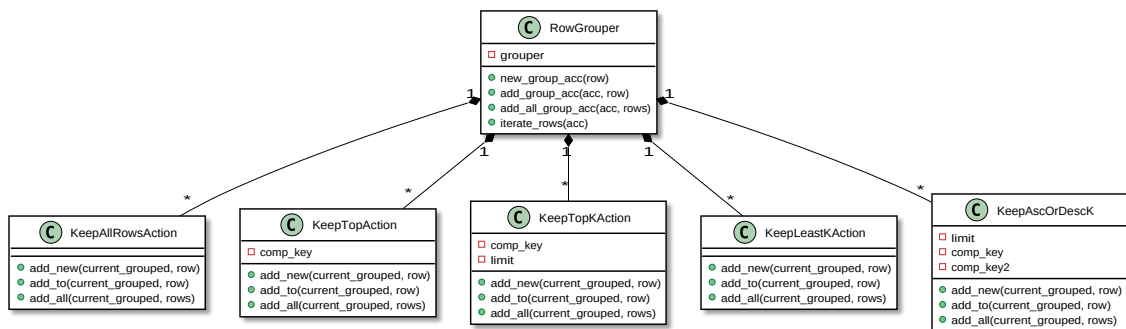
Figura 5: Diagrama de clases del nodo de agrupamiento
