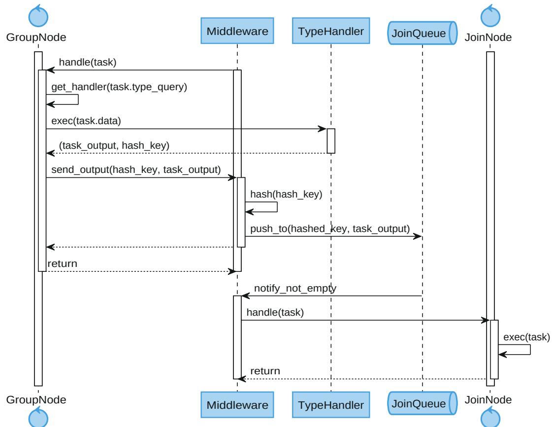
Figura 17: Diagrama de secuencia: Group Node
