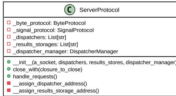
Figura 10: Diagrama de clase del protocolo del servidor
