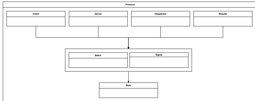
Figura 19: Paquete de protocolos
