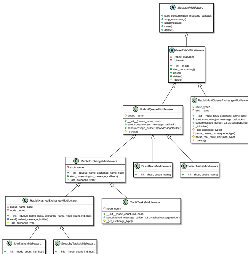
Figura 3: Diagrama de clases de la jerarquía del middleware
