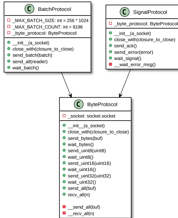
Figura 13: Diagrama de clases de los protocolos de bajo nivel
