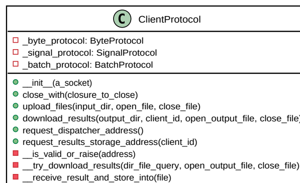
Figura 9: Diagrama de clase del protocolo del cliente
