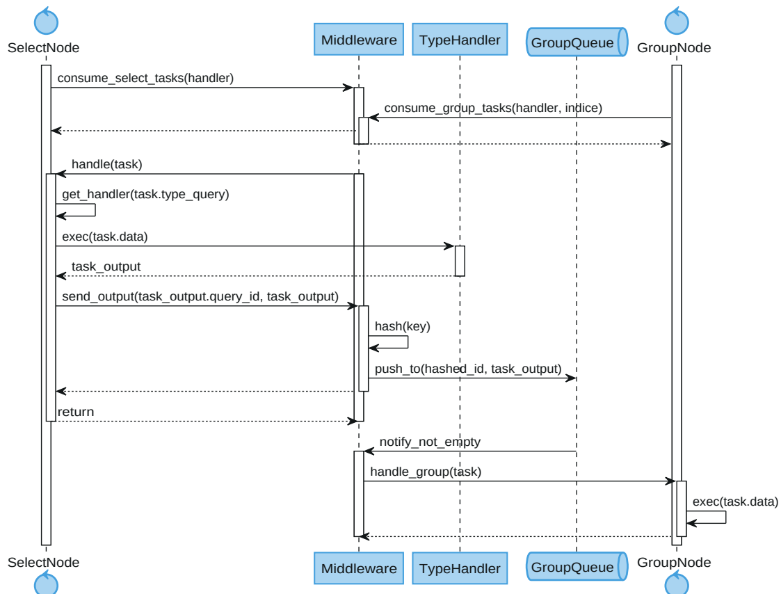
Figura 16: Diagrama de secuencia: Select Node
