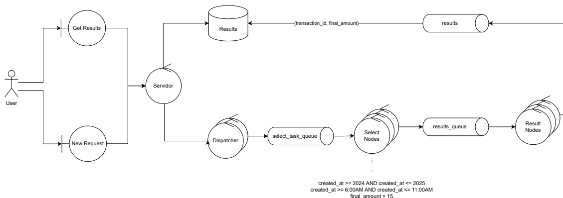
Figura 22: Diagrama de robustez consulta 1°
