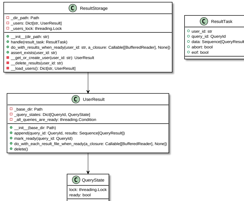
Figura 8: Diagrama de clases del almacenamiento de resultados
