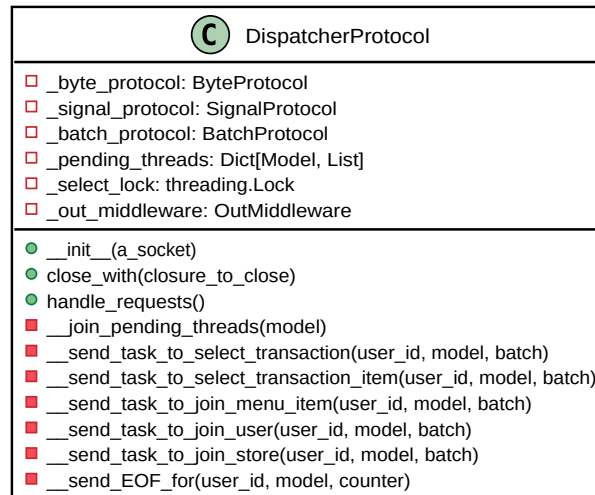
Figura 11: Diagrama de clase del protocolo del dispatcher
