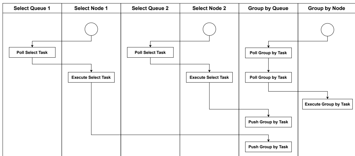
Figura 15: Diagrama de actividades: Selección paralela
