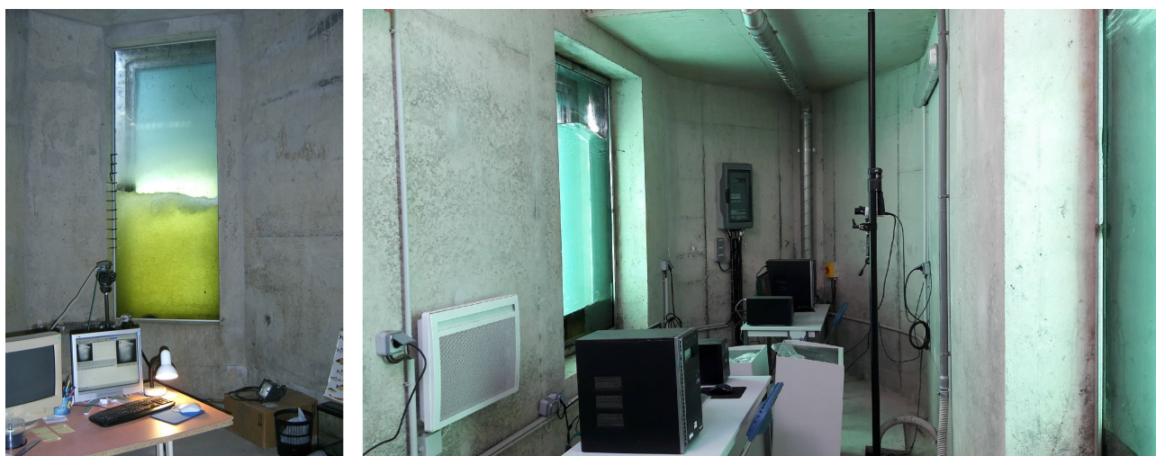
FIGURE 10 – Chambres de vidéo-comptage de la station de contrôle des migrations du barrage de Poses - Amfreville-sous-les-Monts. A gauche, chambre de la rive gauche ; à droite, chambre de la rive droite
