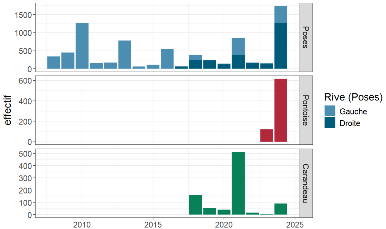
FIGURE 30 – Evolution interannuelle des effectifs d’anguille jaune recensés sur les STACOMI du bassin Seine. Les individus dévalants (codés en ”-1”) sont transformés en valeur positive afin de mieux représenter le volume des anguilles ayant transité par les passes à poissons. Les axes des ordonnées n’ont pas la même échelle.
