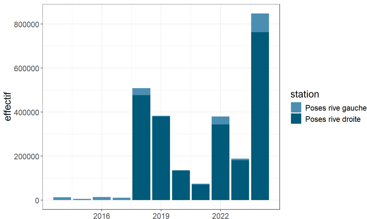
FIGURE 26 – Evolution interannuelle des effectifs des anguilles capturées dans les passes pièges du barrage de Poses - Amfreville-sous-les-Monts
